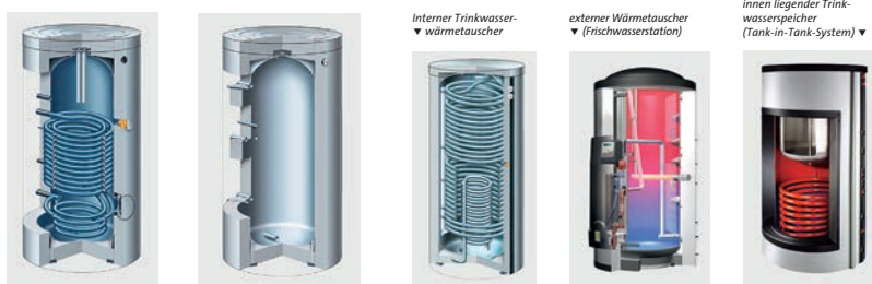
Trinkwarm- wasserspeicher
